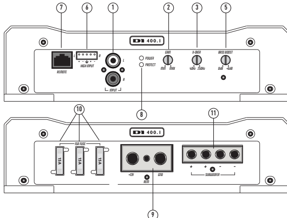
D1 400.1 Mono Amplifier
